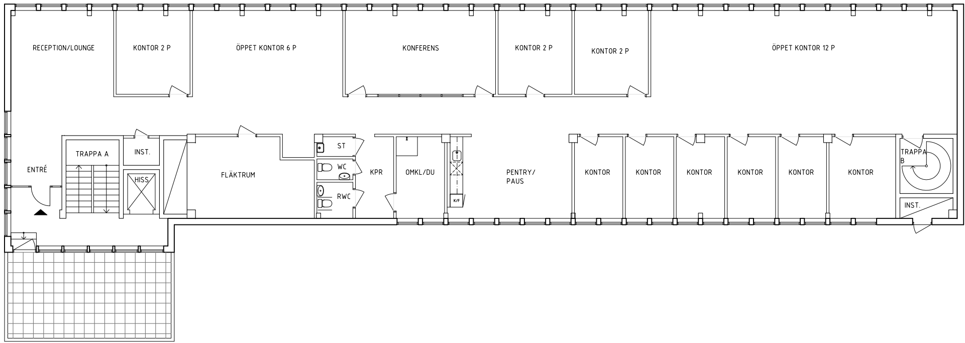
PLAN 4, VÅN. 4 TRAPPOR
