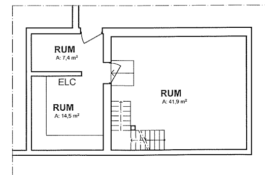
KÄLLARPLAN BRUKSAREA 67,0 m 2
