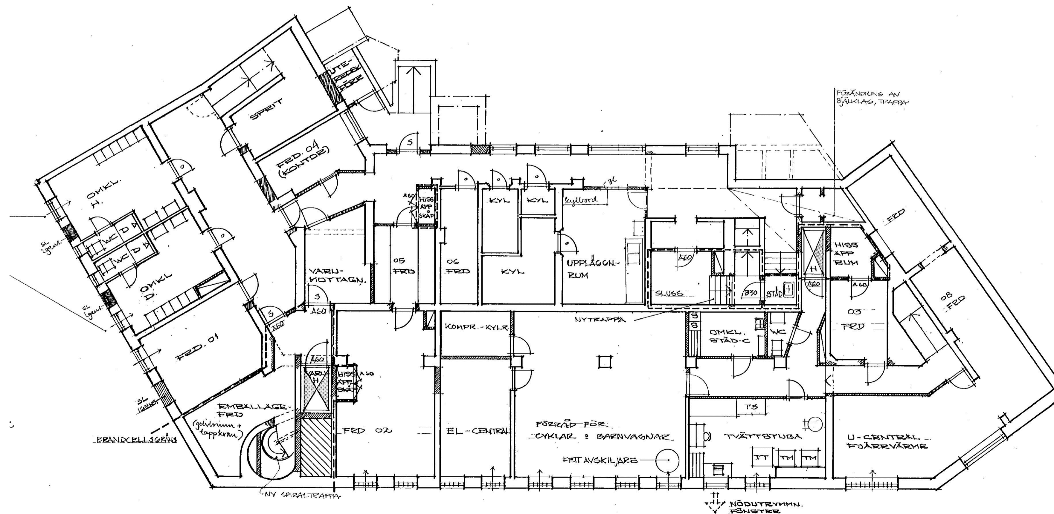
KÄLLARPLAN
