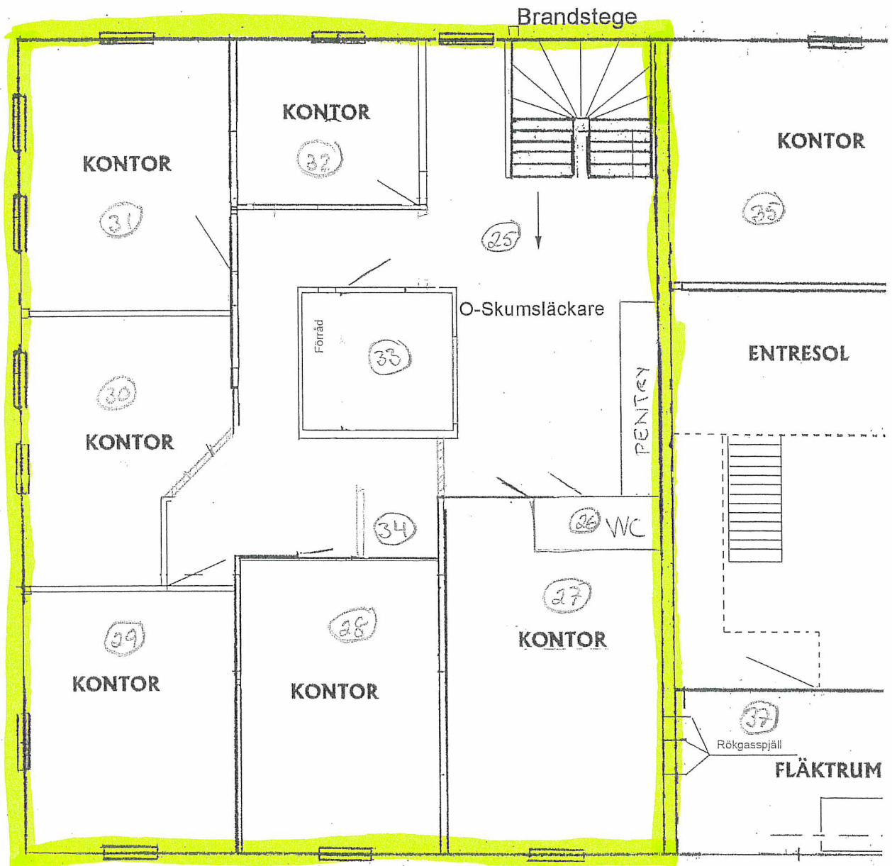
Våningsplan 1:100
